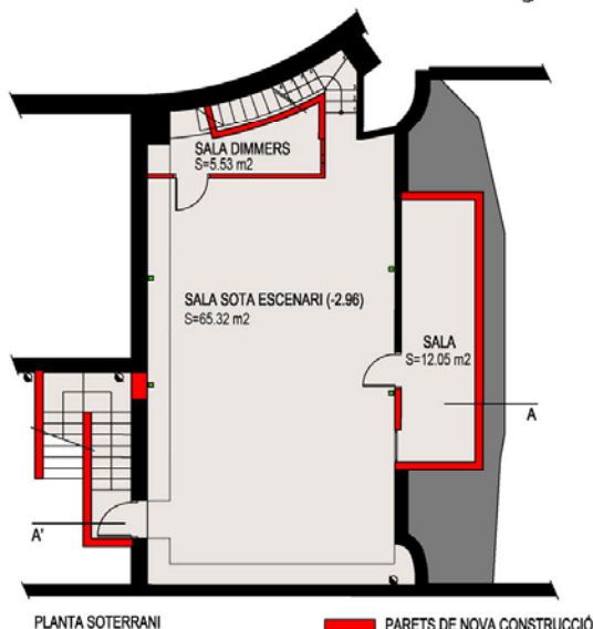
PLANTA SOTERRANI
