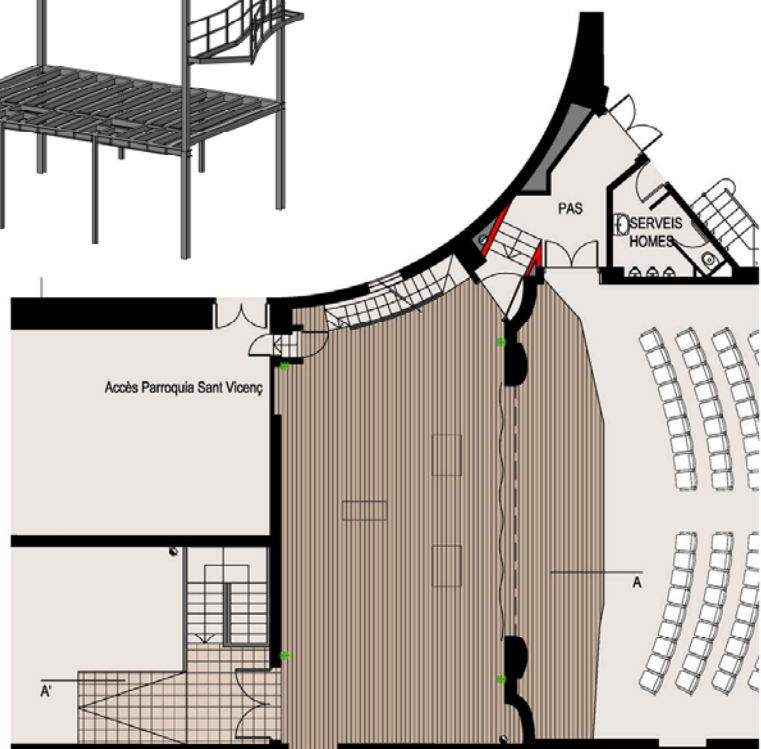
PLANTA BAIXA
