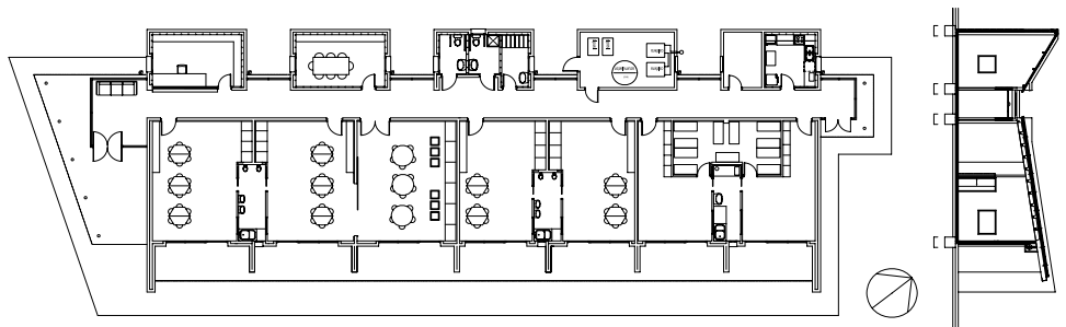
PLANTA BAIXA
