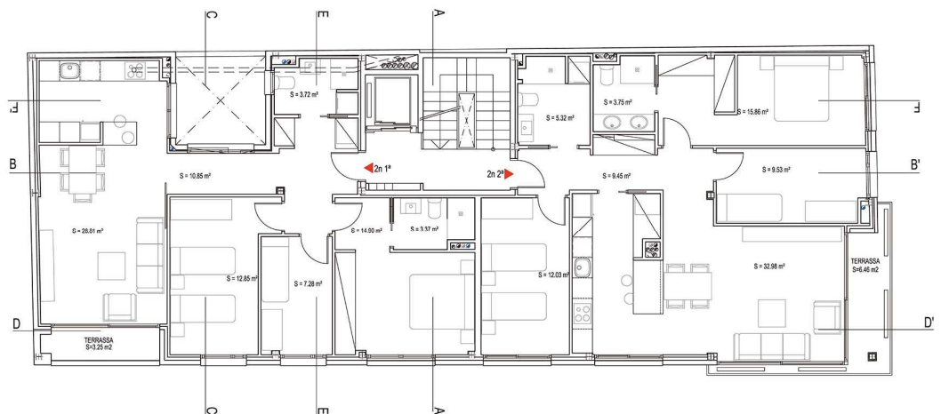
PLANTA SEGONA
