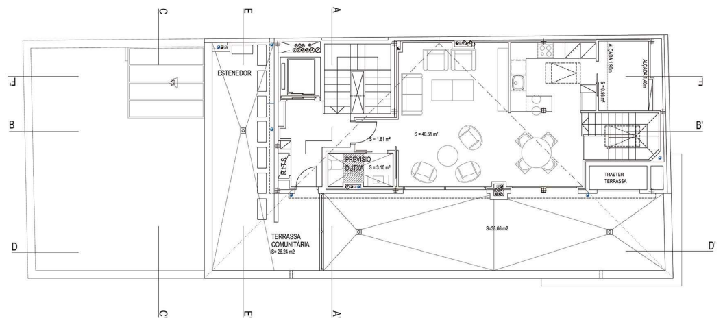
PLANTA SOTACOBERTA
